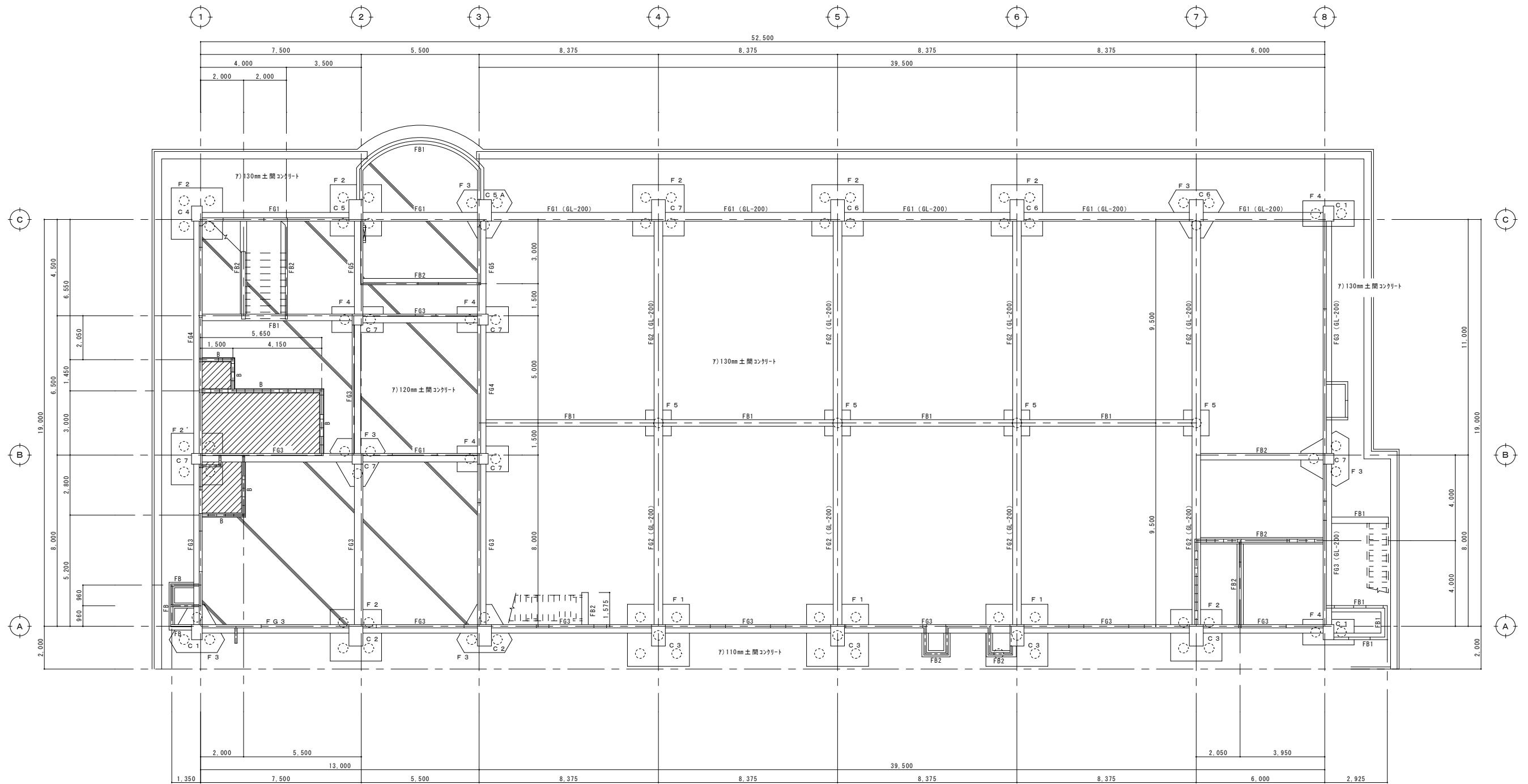
基礎伏図 A3:S=1:200 A1:S=1:100
