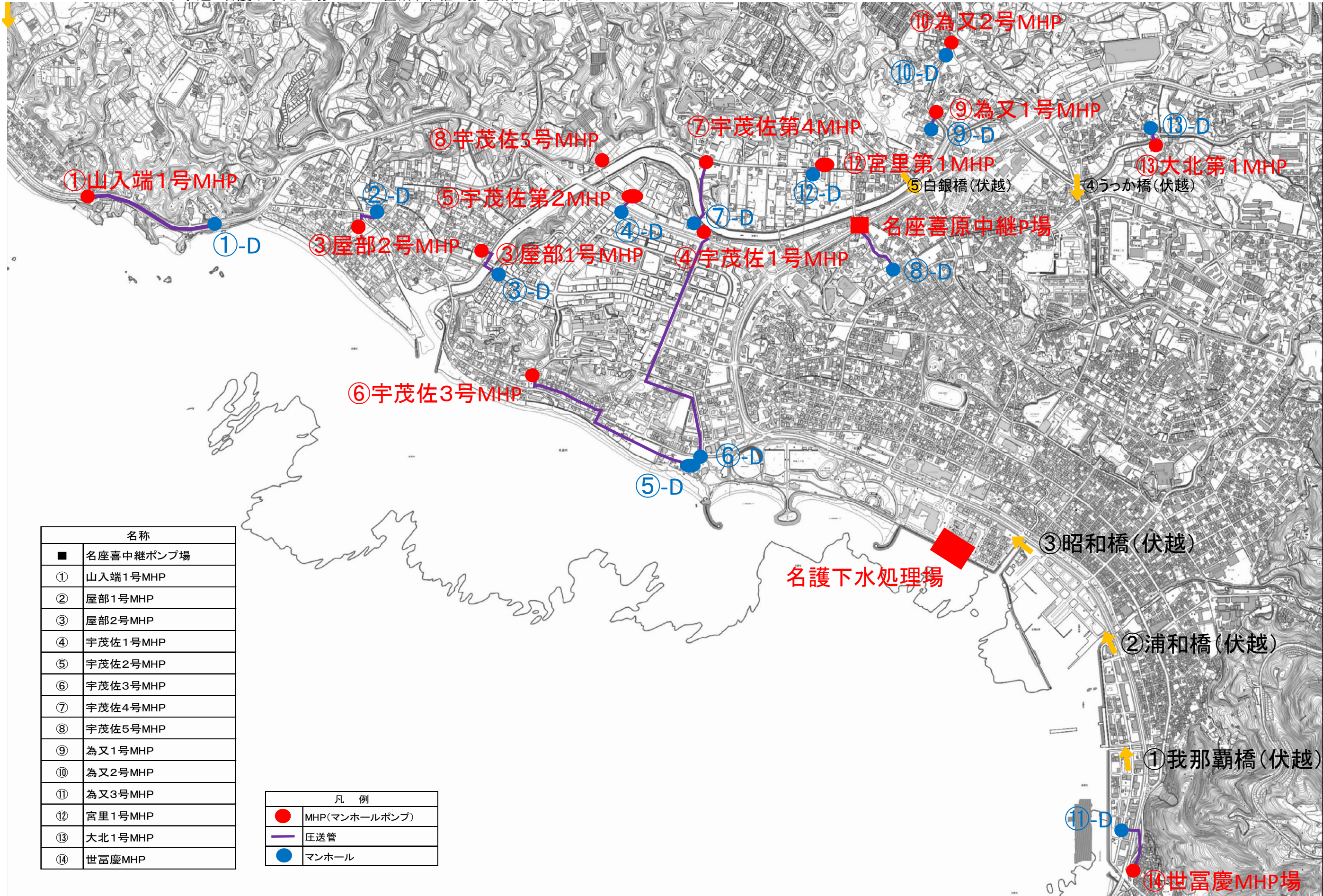
公共下水道 名護下水処理場 MHP14箇所、中継P場1箇所 位置図(1)
