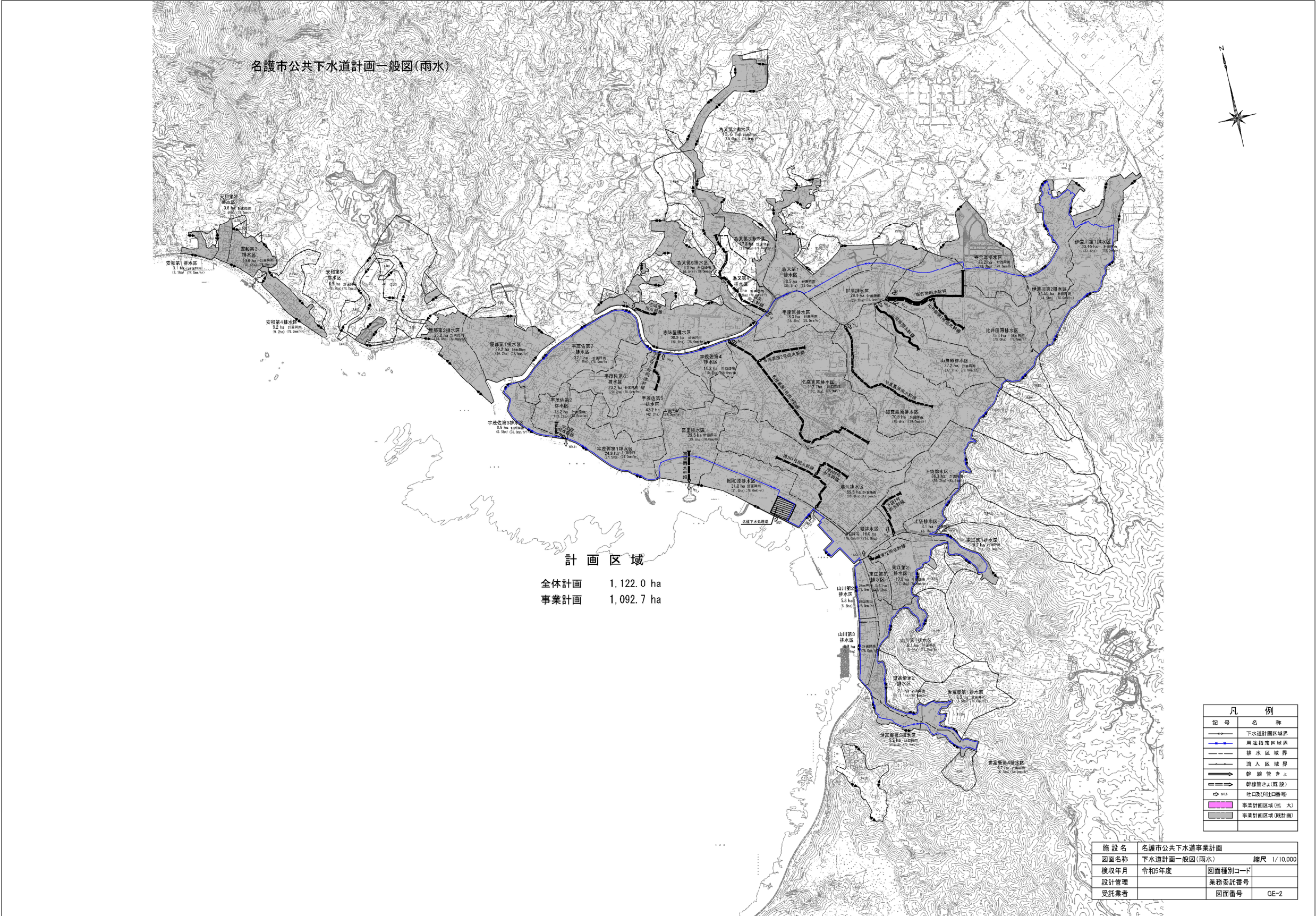
図 2 下水道計画一般図(雨水)_名護処理区
