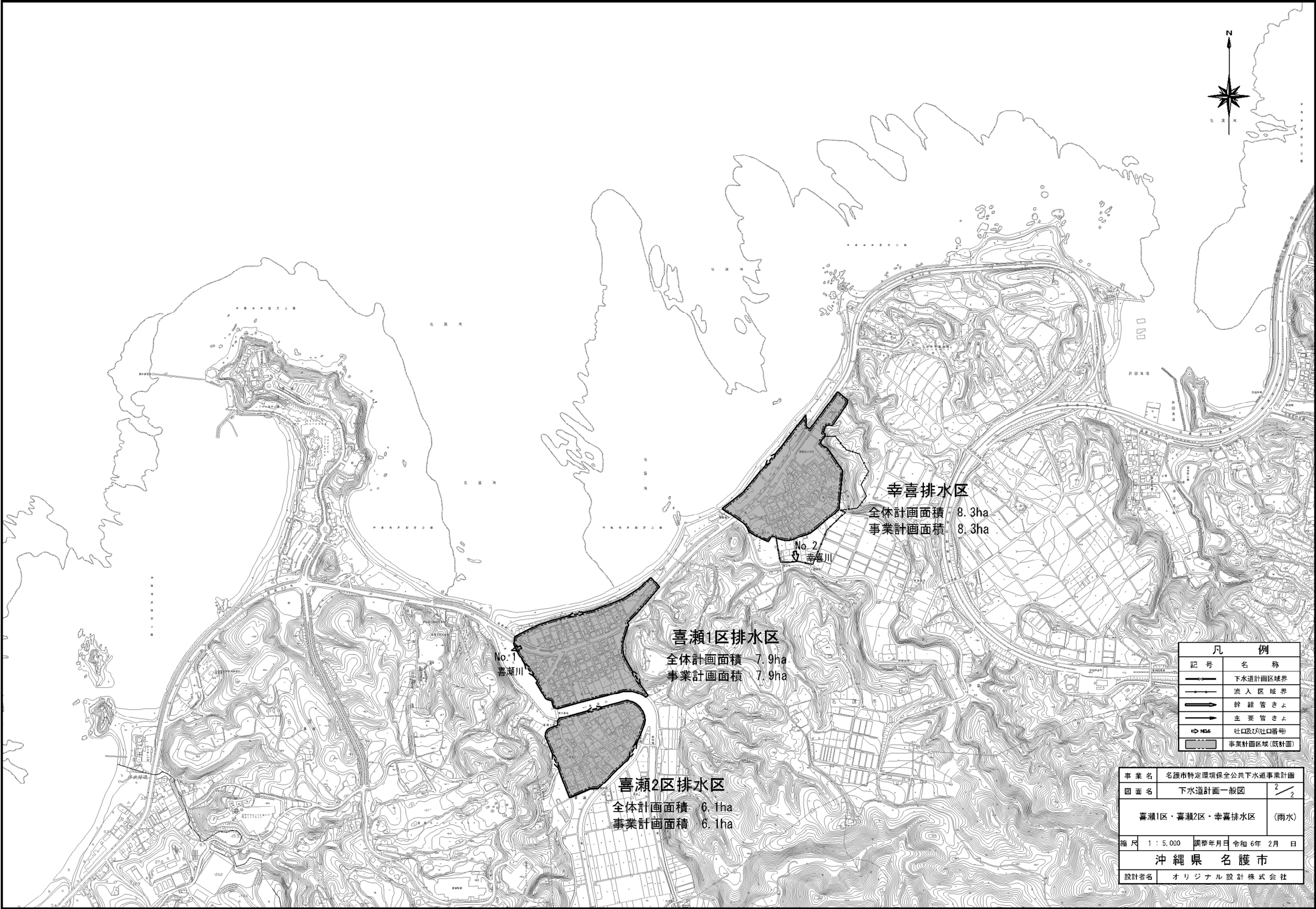
図 4 下水道計画一般図（雨水）_喜瀬・幸喜処理区
