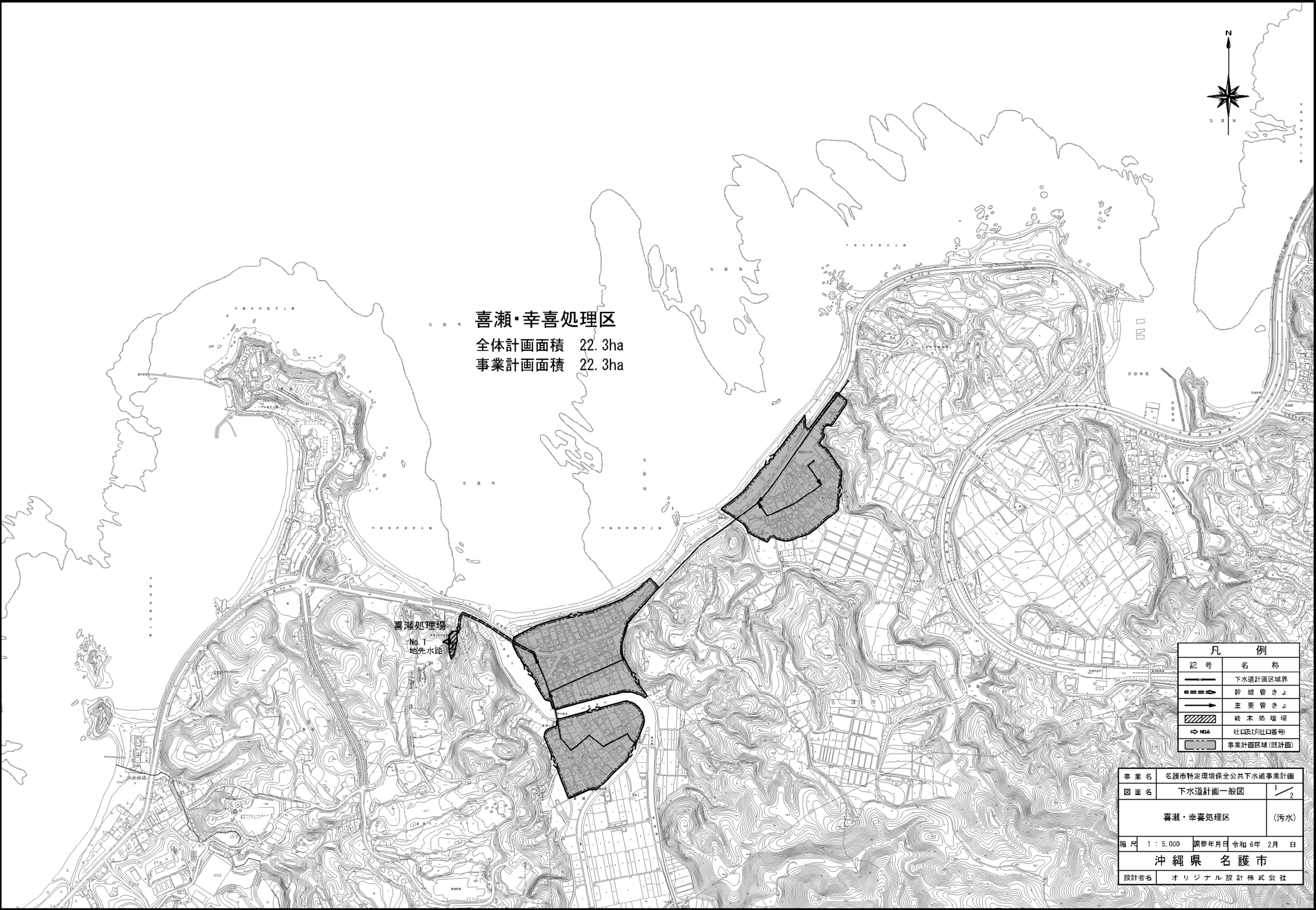
図3 下水道計画一般図（汚水）_喜瀬・幸喜処理区
