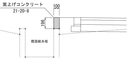
断面図
