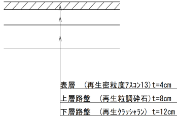
取付道路舗装 S=1/10
