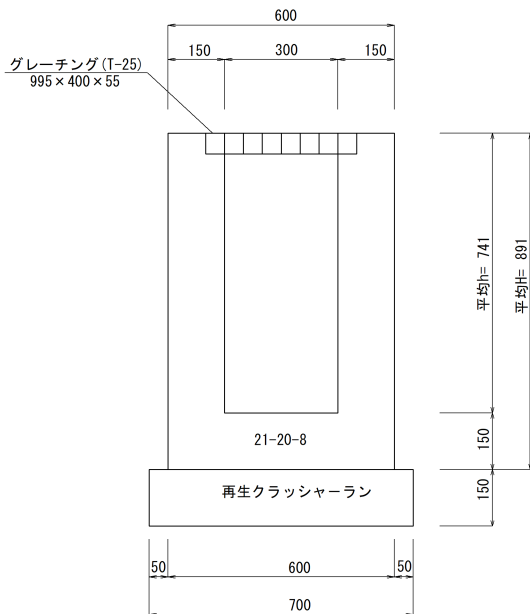
1号横断側溝
