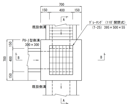
7号集水樹
