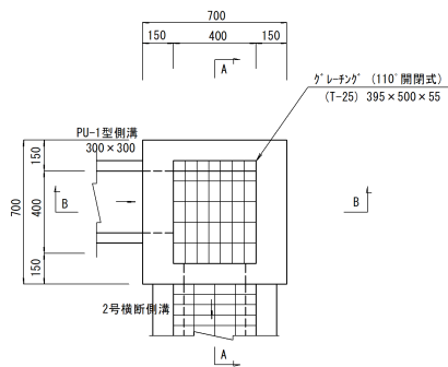
6号集水樹
