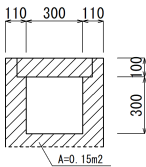
既設側溝撤去 S=1/20
