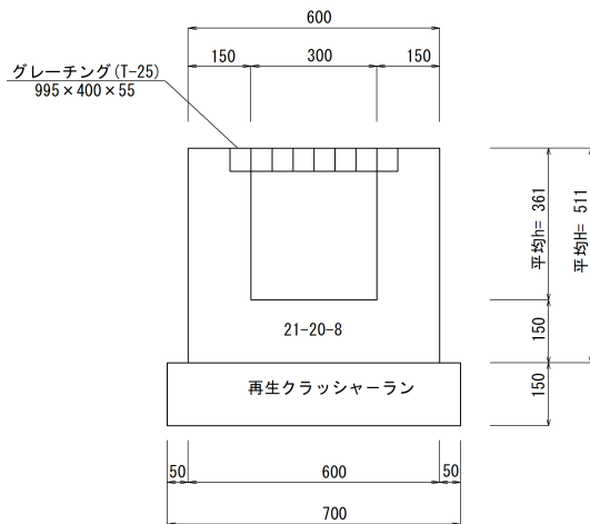
2号横断側溝
