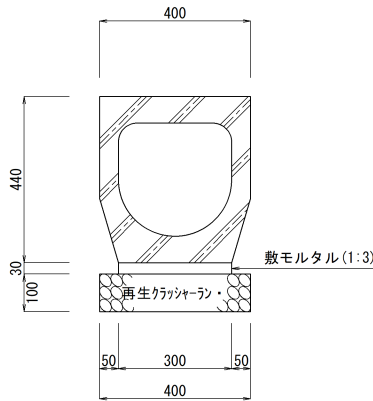
1型埋設管
