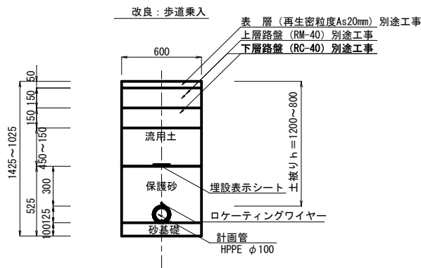
⑨－３－１型管土工
