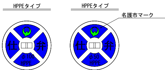
仕切弁筐蓋
