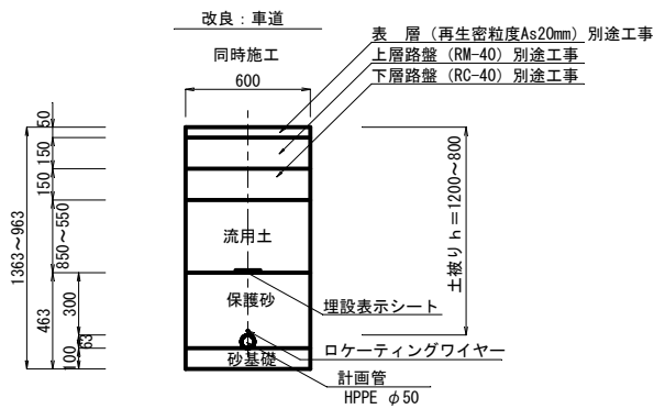
⑧－３－１型管土工
