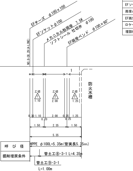
防火水槽
