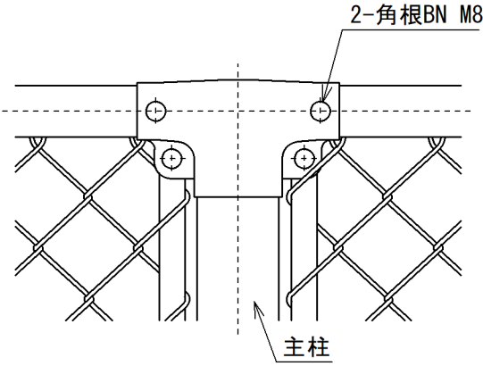
B 部取付図 S=1:5
