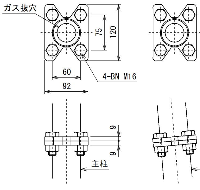
C 部取付図 S=1:5
