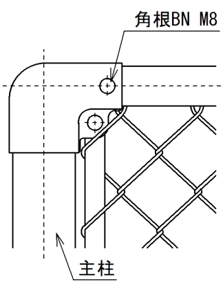
A 部取付図 S=1:5
