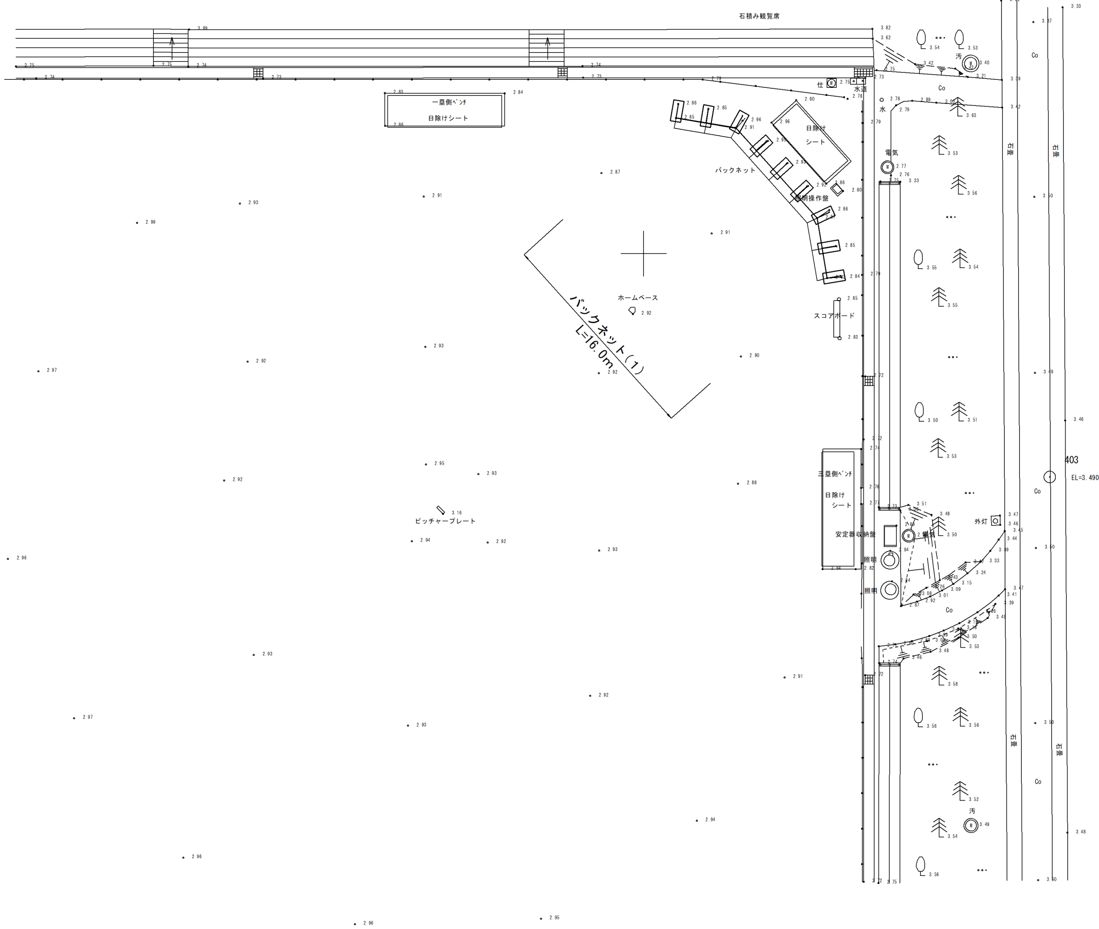
計画平面図（１） S=1:250
