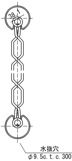
胴縁に金網取付断面図 S=1:3
