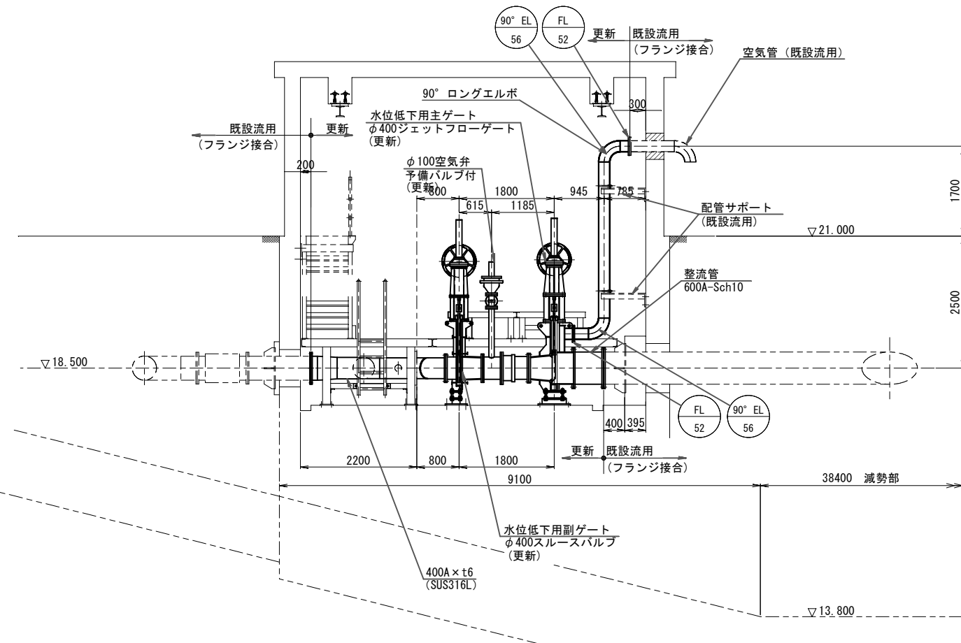
側面図
