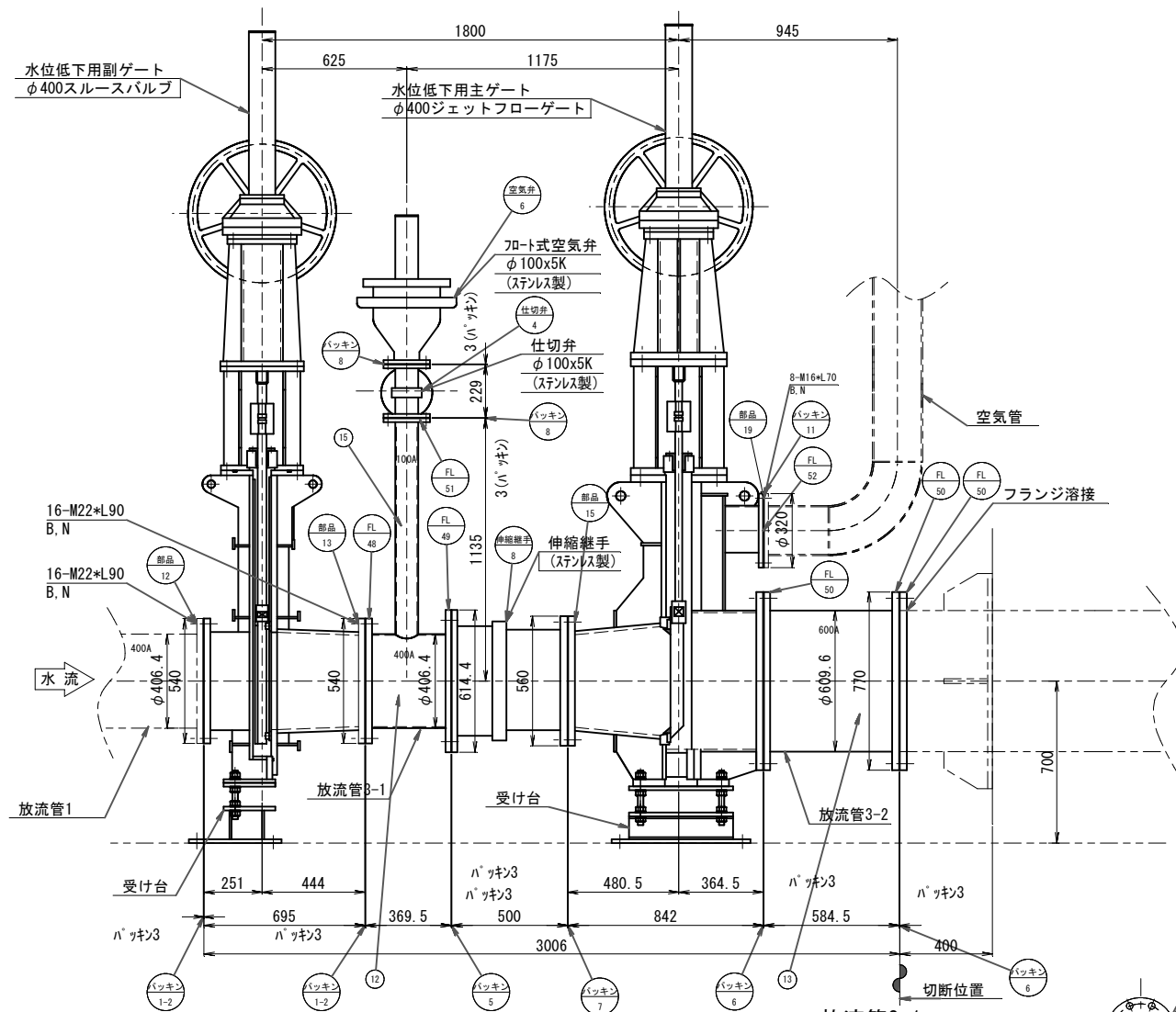
放流管3-1 S=1:10
