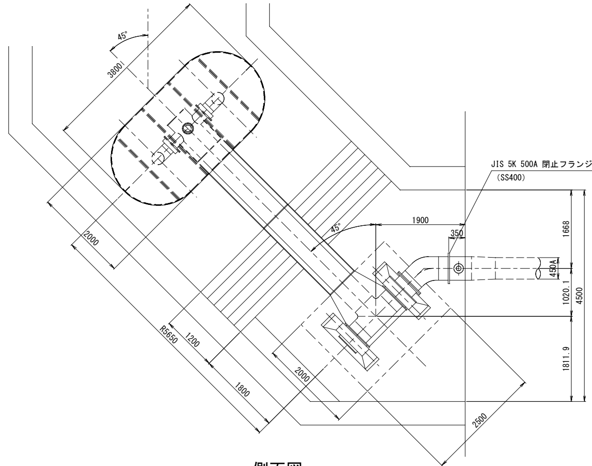
側面図
