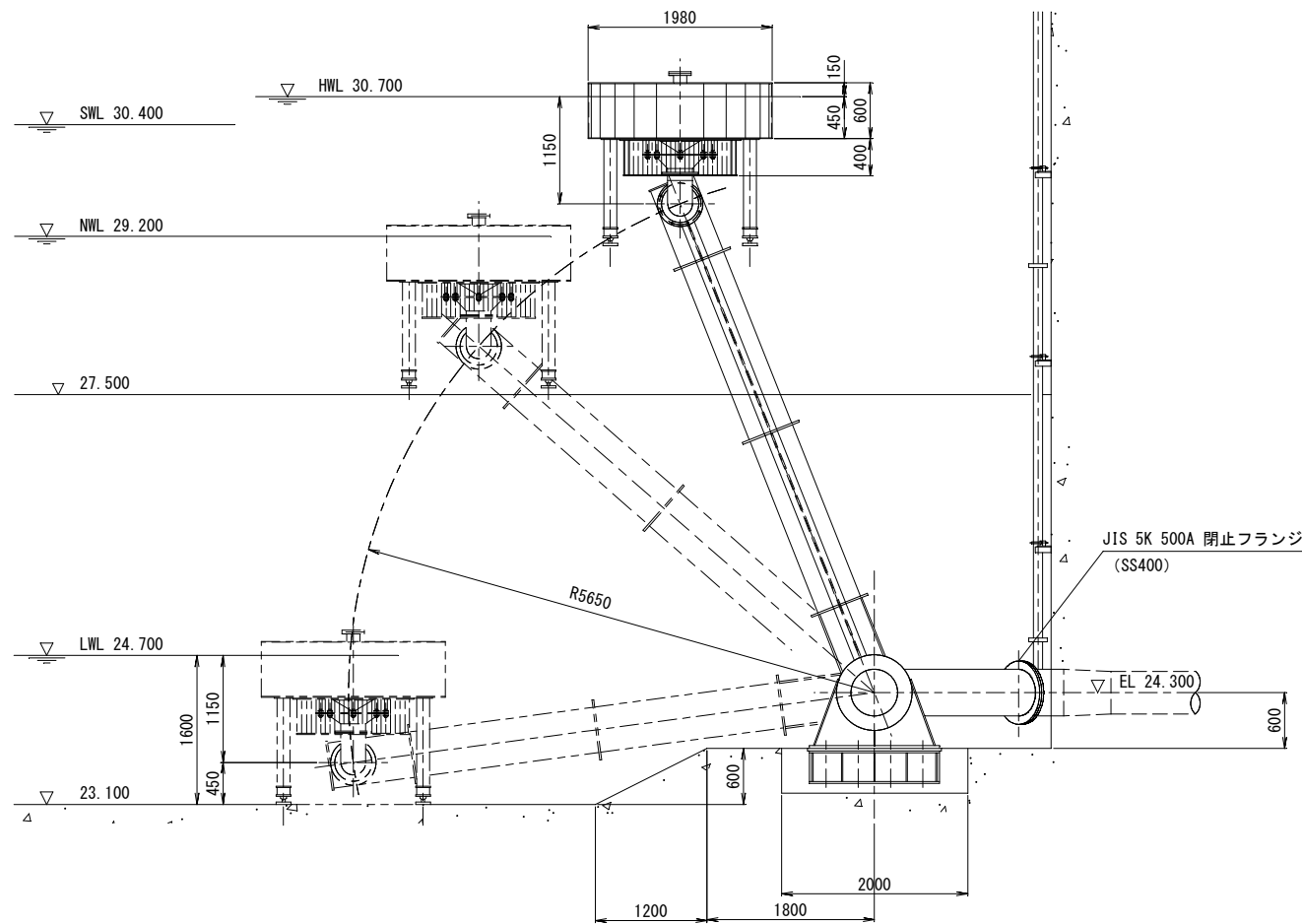
側面図
