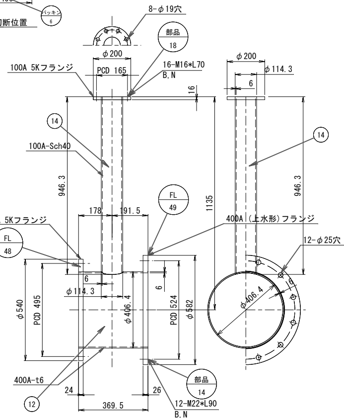
放流管3-1 S=1:10
