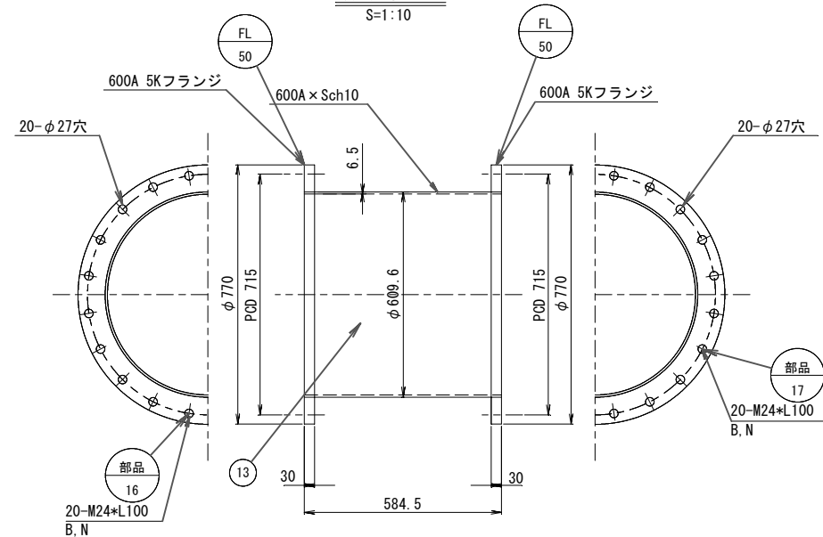
放流管3-2 S=1:10
