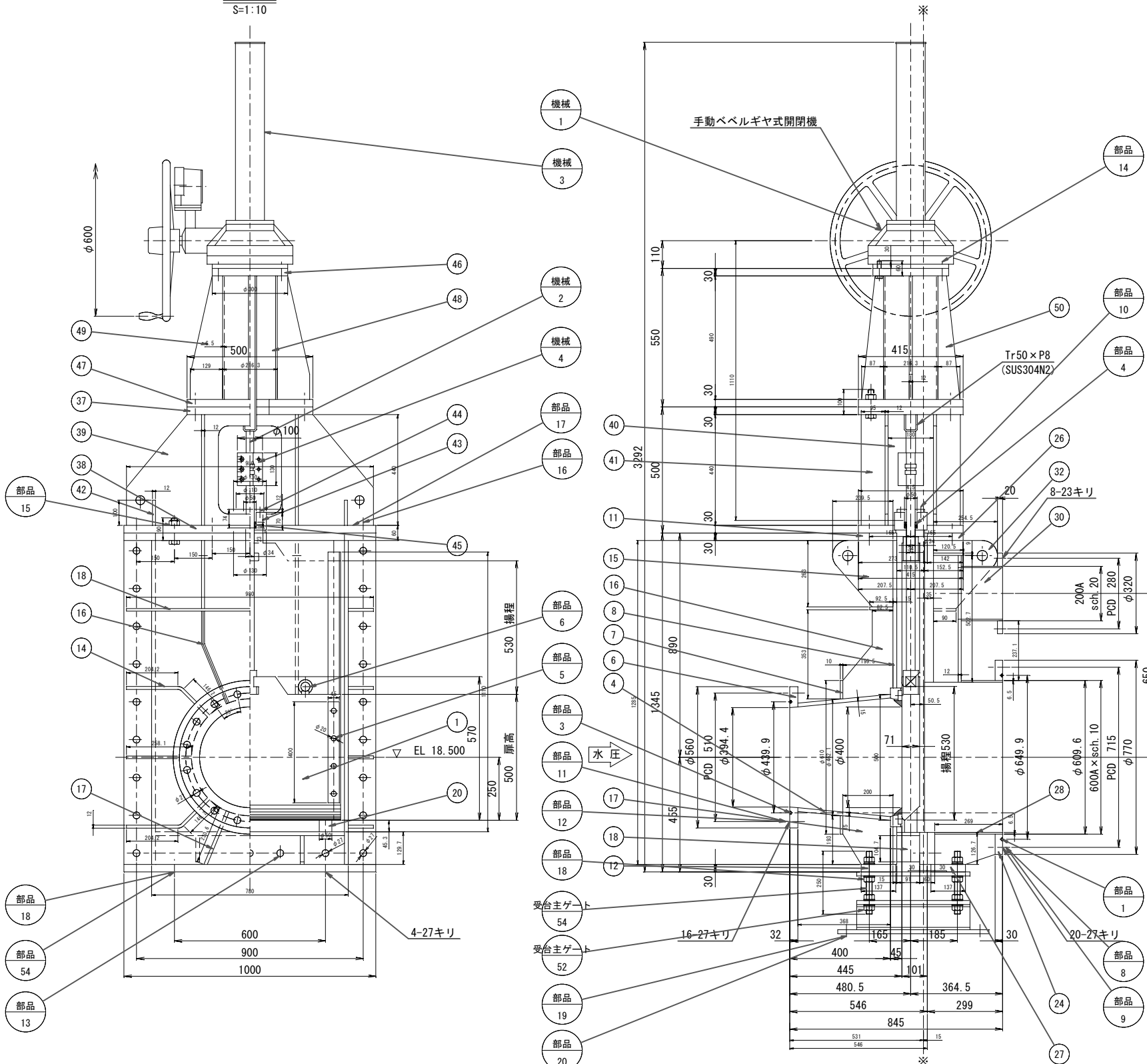
正面図 S=1:10
