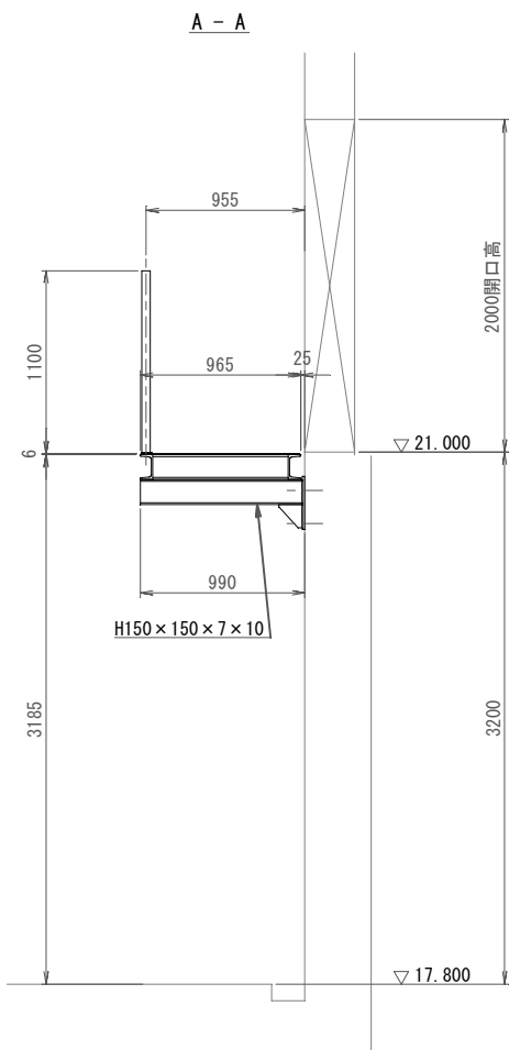
詳細図
