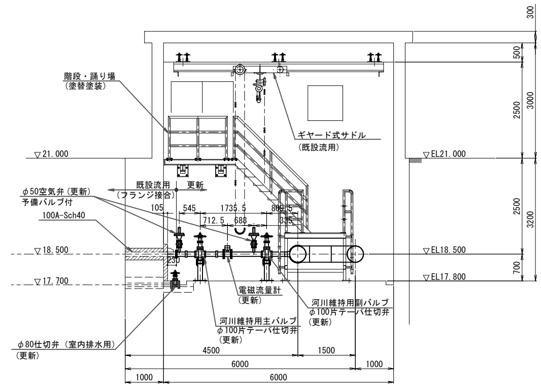
側面図
