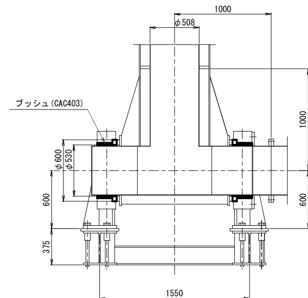
詳細図B
