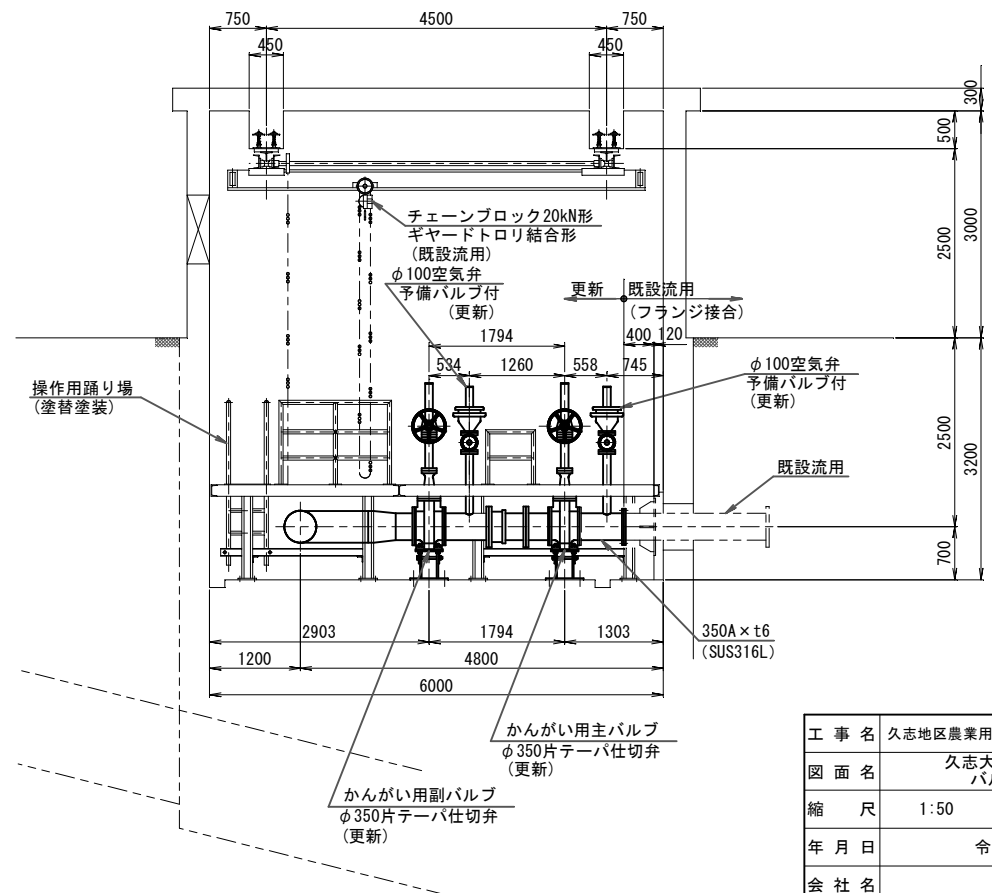
側面図
