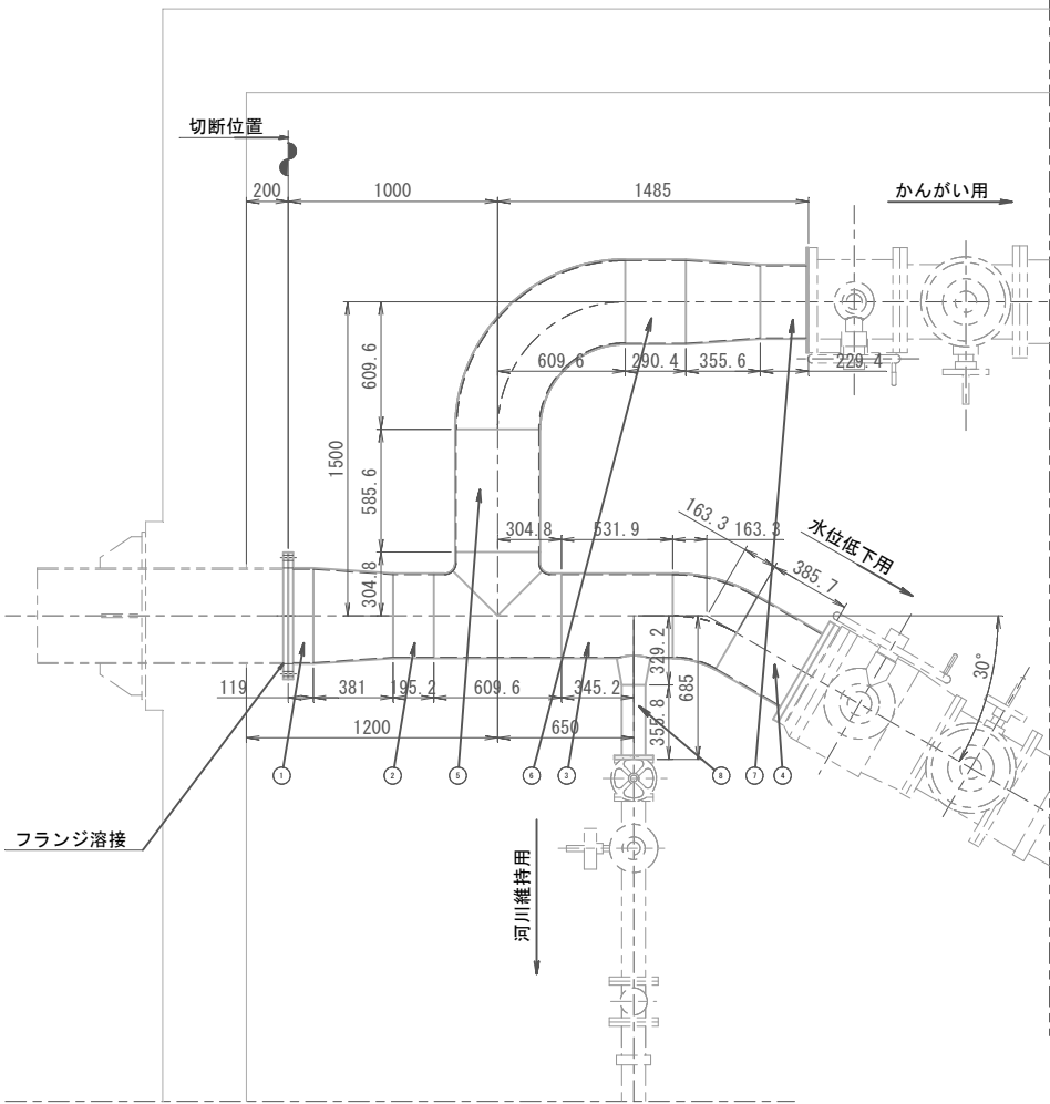
配置図 S=1:20
