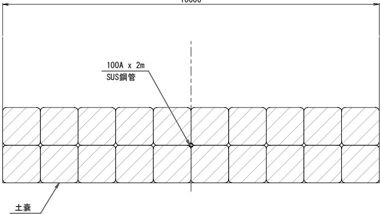
詳細図A
