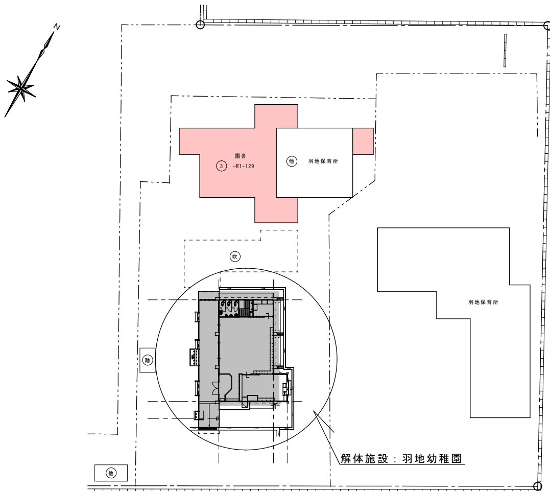
配置図
