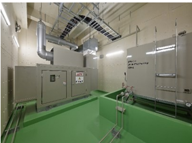
3階 発電機室
