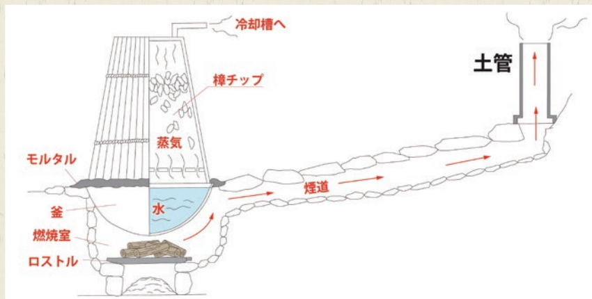
樟脳製造の予想模式図
