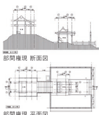
部間権現 平面図
