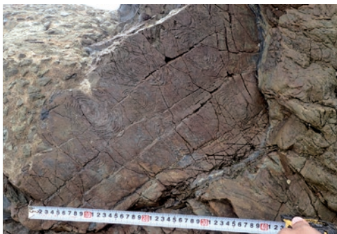
栈橋遺構付近で確認された生痕化石
